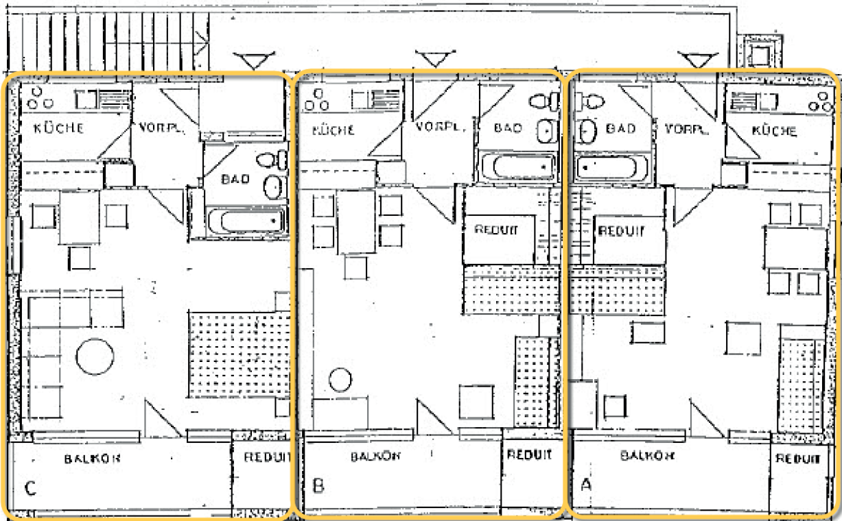
3 Wohnungen pro Haus und Etage
